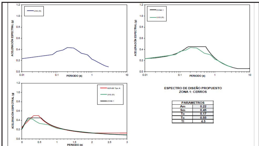
Figura 3: Espectros uniformes de amenaza en roca y espectro de diseño establecido para la microzona 1 de Santiago de Cali.
