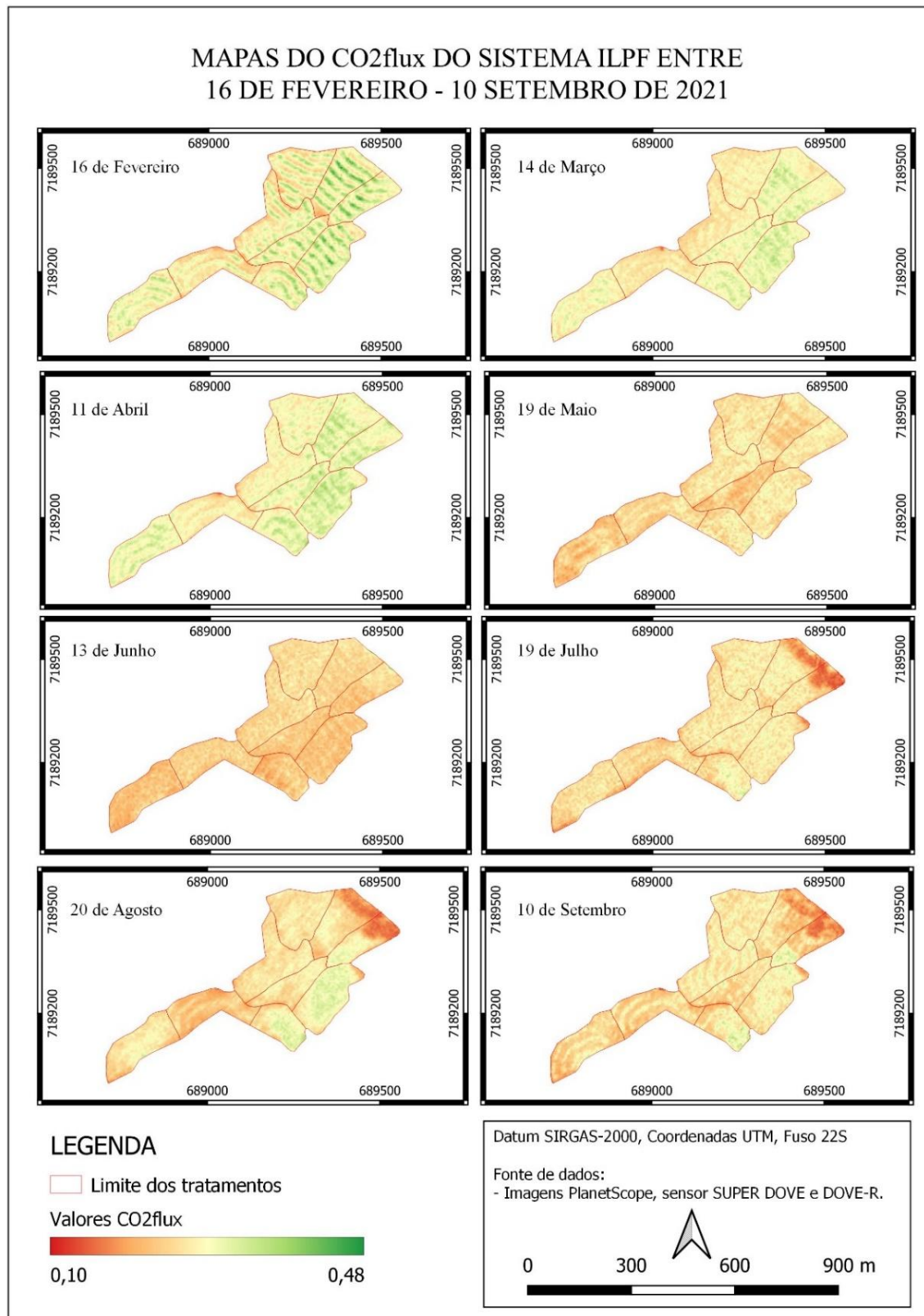
Figura 5. MAPAS DO CO 2 FLUX DA ÁREA DE ESTUDO ENTRE OS MESES DE FEVEREIRO E SETEMBRO DE 2021
