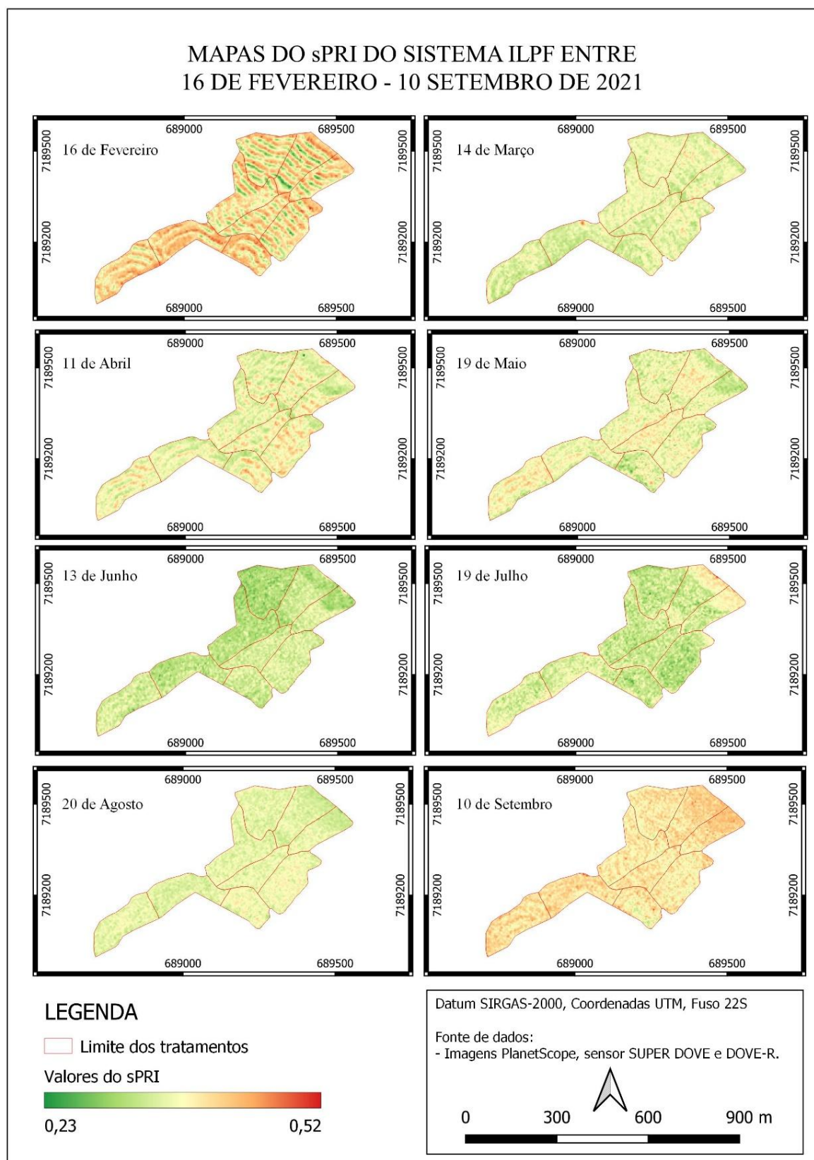
Figura 6. MAPAS DO sPRI DA ÁREA DE ESTUDO ENTRE OS MESES DE FEVEREIRO E SETEMBRO DE 2021
