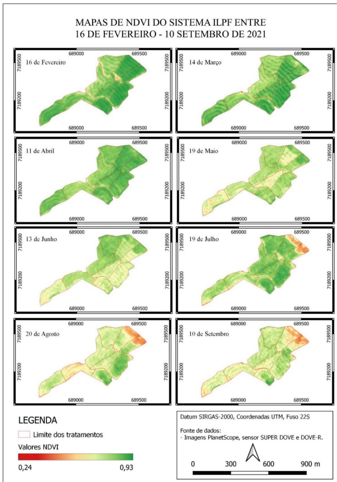
Figura 4. MAPAS DE NDVI DA ÁREA DE ESTUDO, ENTRE OS MESES DE FEVEREIRO E SETEMBRO DE 2021
