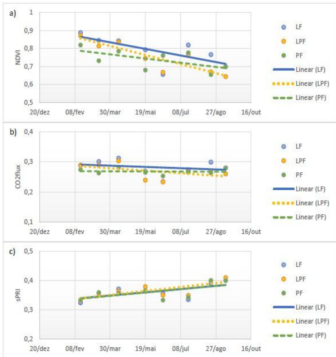
Figura 2. VARIAÇÃO TEMPORAL DOS VALORES MÉDIOS DE NDVI, CO 2 flux e sPRI - NÍVEL DE PIXEL (PIXELS COINCIDENTES COM A LOCALIZAÇÃO DAS ÁRVORES). AS LINHAS (LINEAR) REPRESENTAM A REGRESSÃO LINEAR PARA CADA TRATAMENTO
