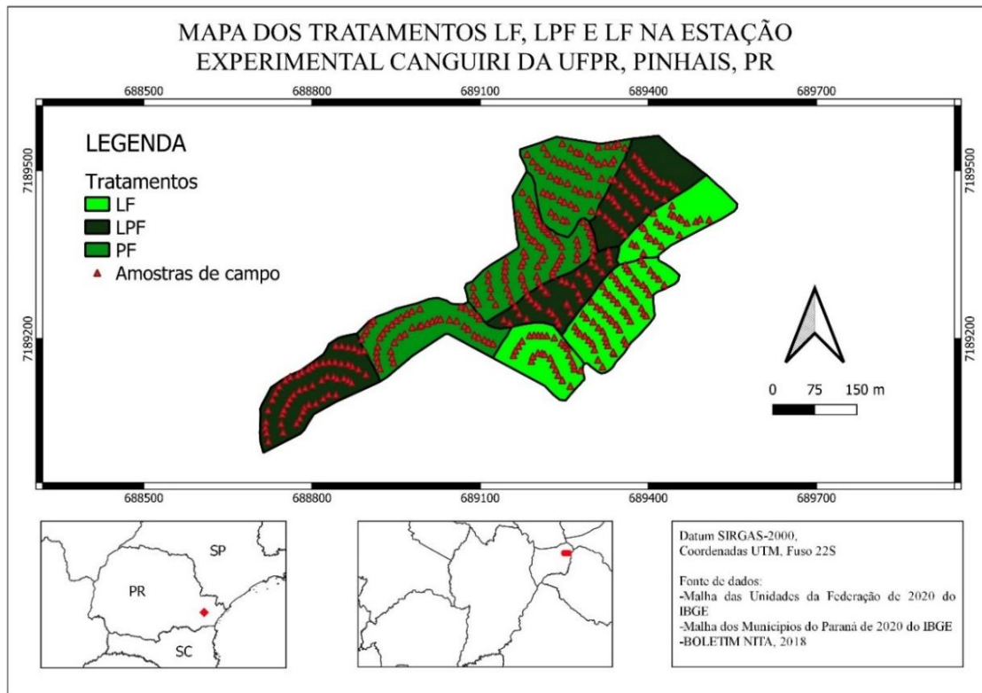
Figura 1. MAPA DE LOCALIZAÇÃO DOS TRATAMENTOS LF, LPF E PF NA ESTAÇÃO EXPERIMENTAL CANGUIRI DA UFPR, EM PINHAIS, PR
