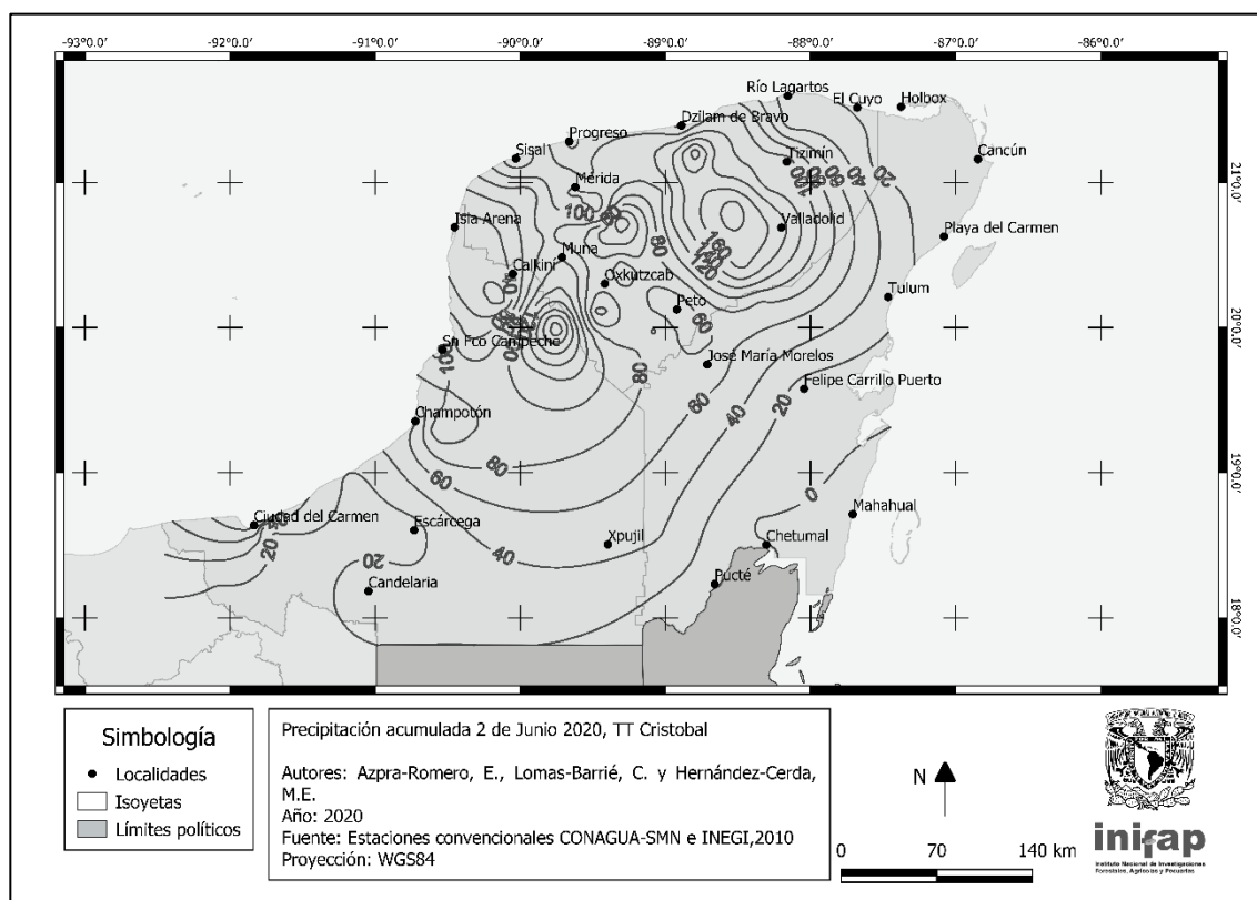
Figura 14. Precipitaciones (mm) del 2 de junio de acuerdo a los datos de las estaciones convencionales de superficie, en la Península de Yucatán
