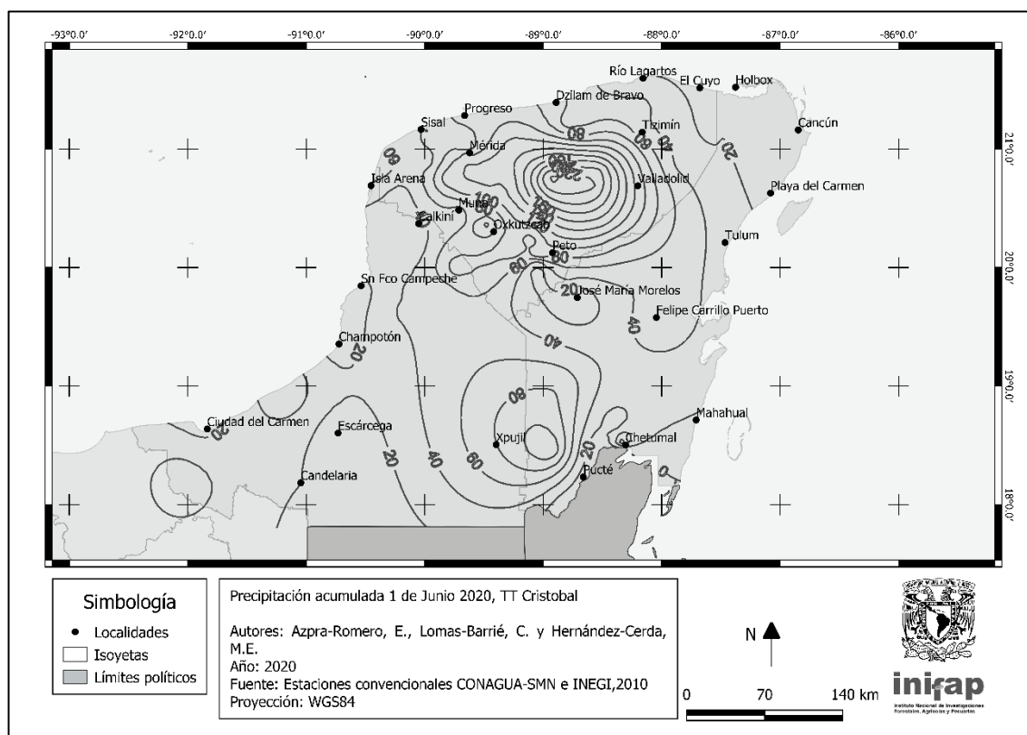
Figura 13. Precipitaciones (mm) del 1 de junio de acuerdo a los datos de las estaciones convencionales de superficie, en la Península de Yucatán
