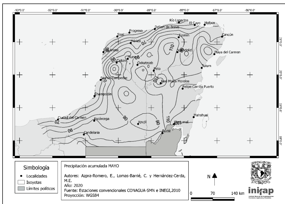
Figura 5. Precipitación media acumulada (mm) del mes de mayo para la Península de Yucatán
