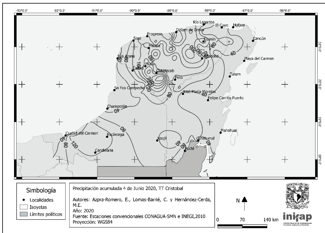
Figura 16. Precipitaciones (mm) del 4 de junio de acuerdo a los datos de las estaciones convencionales de superficie, en la Península de Yucatán
