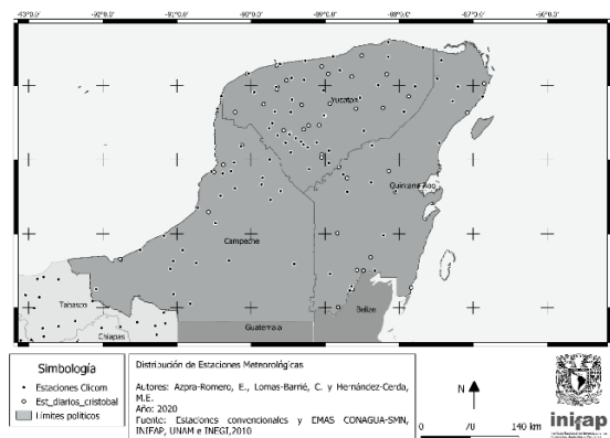
Figura 2. Localización de las estaciones meteorológicas convencionales y automatizadas.
