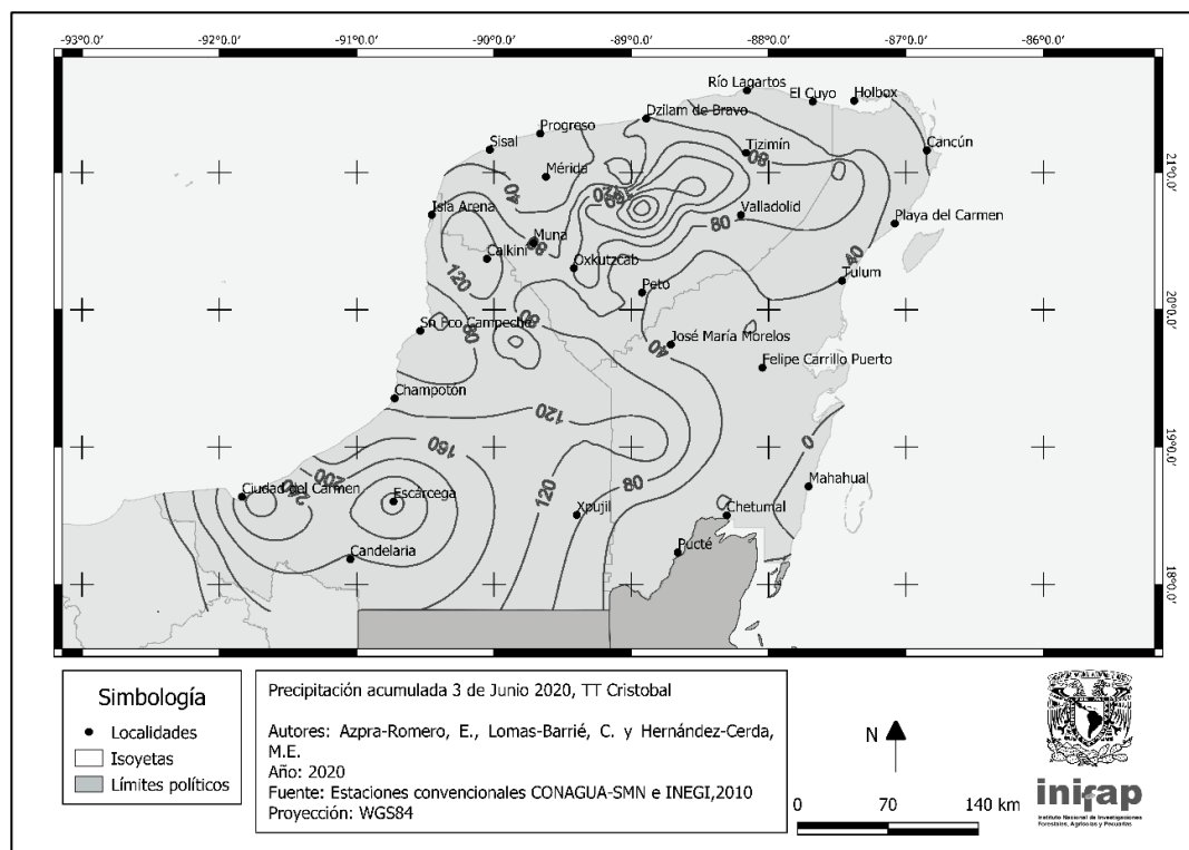
Figura 15. Precipitaciones (mm) del 3 de junio de acuerdo a los datos de las estaciones convencionales de superficie, en la Península de Yucatán
