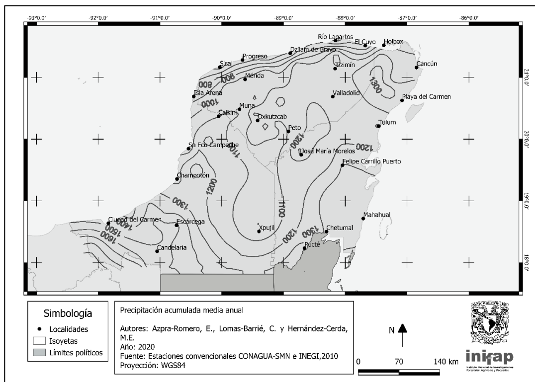
Figura 3. Precipitaciones medias anuales (mm) acumuladas en la Península de Yucatán
