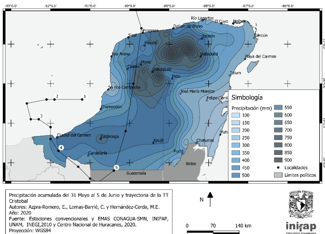
Figura 19. Precipitaciones acumuladas (mm) del 31 de mayo al 5 de junio de 2020, registradas en las estaciones convencionales y automáticas
