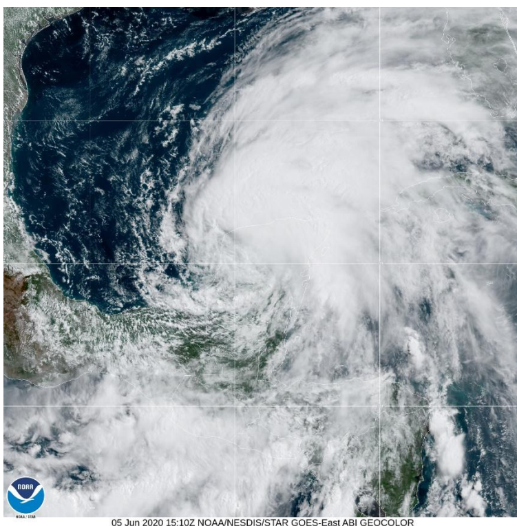
Figura 18. Imagen del satélite GOES 16 composición ABI GEOCOLOR del 5 de junio a las 15:10UTC.
