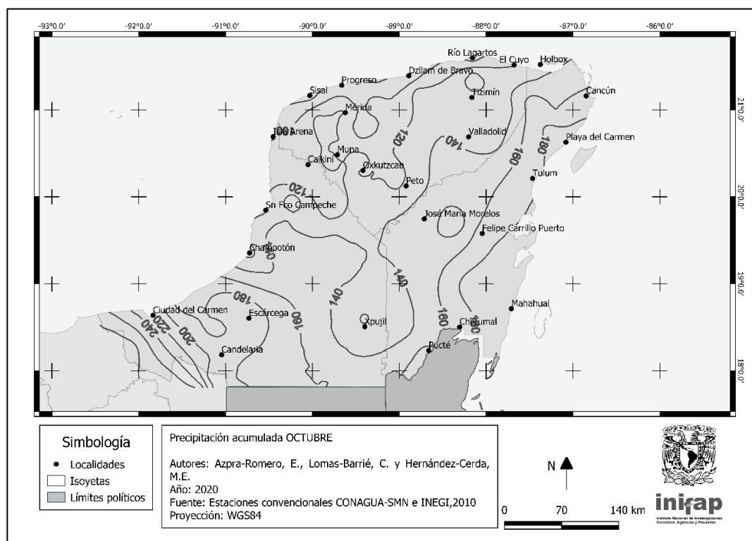
Figura 10. Precipitación media acumulada (mm) del mes de octubre para la Península de Yucatán
