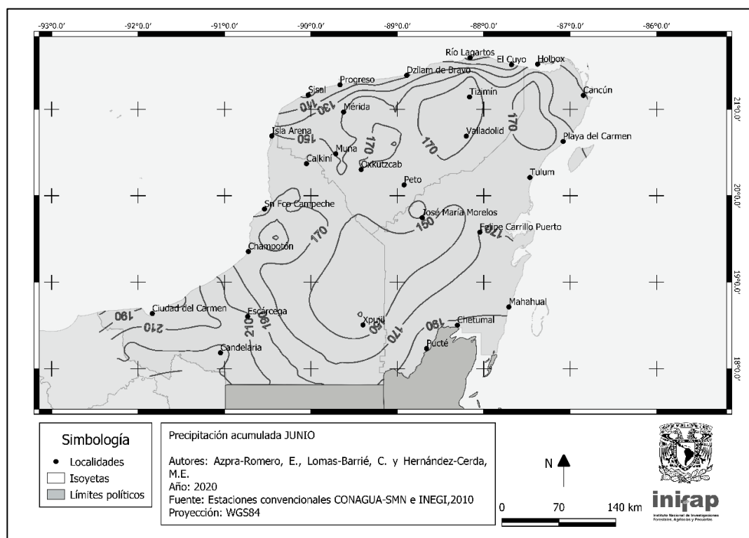
Figura 6. Precipitación media acumulada (mm) del mes de junio para la Península de Yucatán
