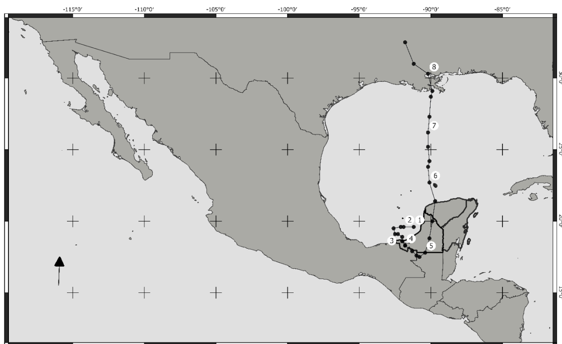
Figura 11. Trayectoria de la TT Cristóbal (01-08 junio, 2020). Los números indican los días del mes de junio.
