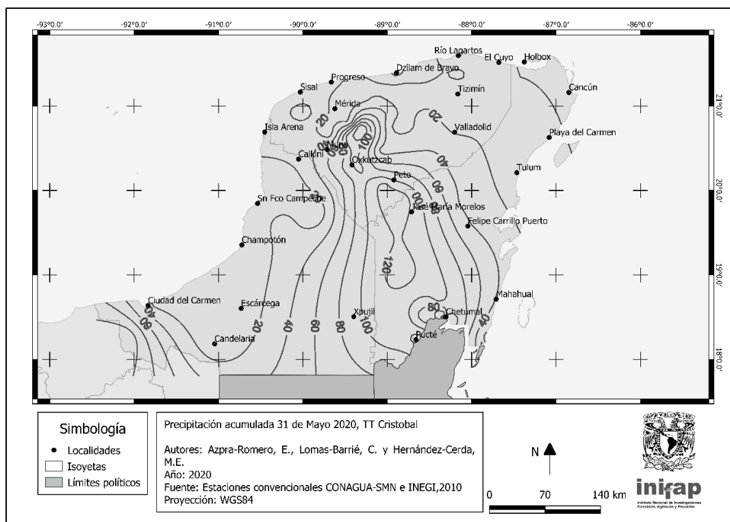
Figura 12. Precipitaciones (mm) del 31 de mayo de acuerdo a los datos de las estaciones convencionales de superficie, en la Península de Yucatán.
