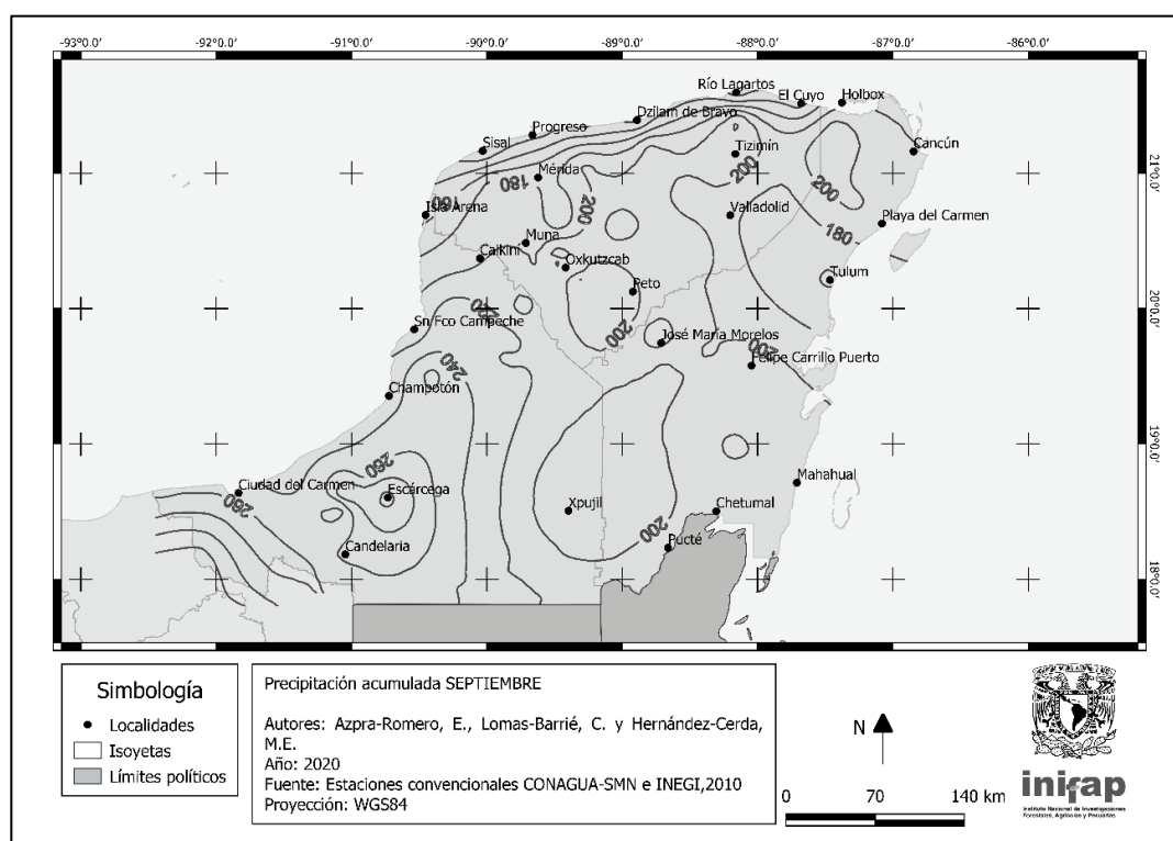
Figura 9. Precipitación media acumulada (mm) del mes de septiembre para la Península de Yucatán.
