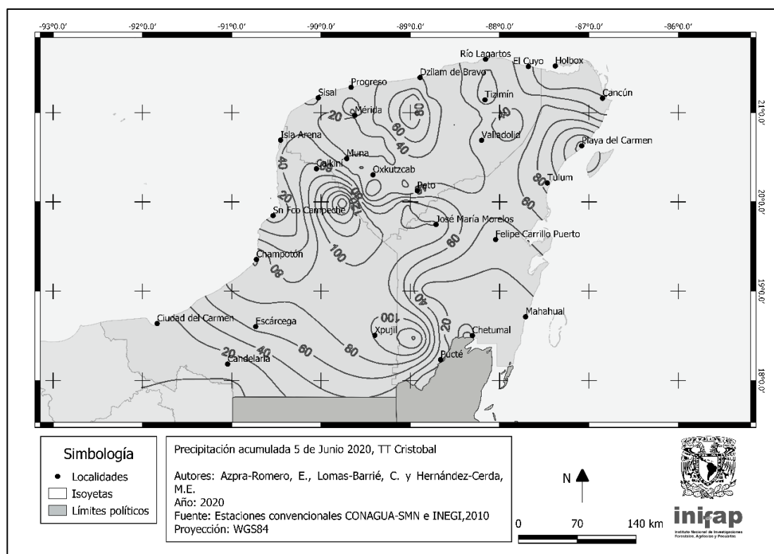
Figura 17. Precipitaciones (mm) del 5 de junio de acuerdo a los datos de las estaciones convencionales de superficie, en la Península de Yucatán
